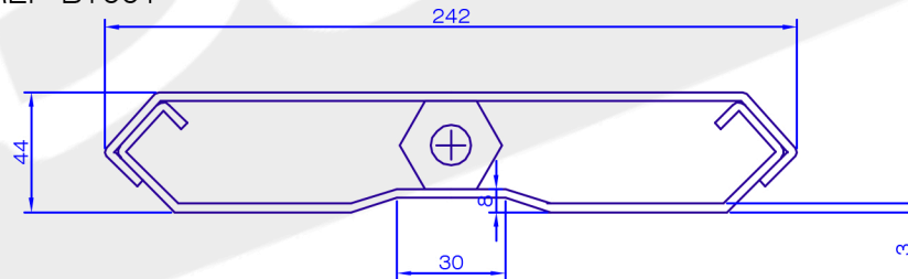
VISTA FRONTAL REF-BT001
